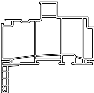
1" FLUSH FIN
